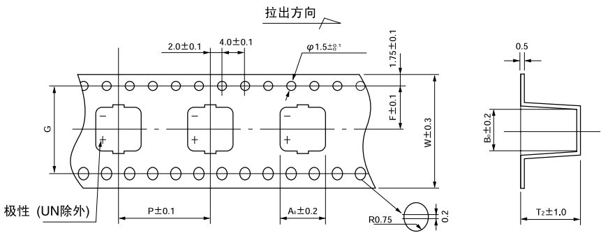
图2 (适用于φ12.5以上)
